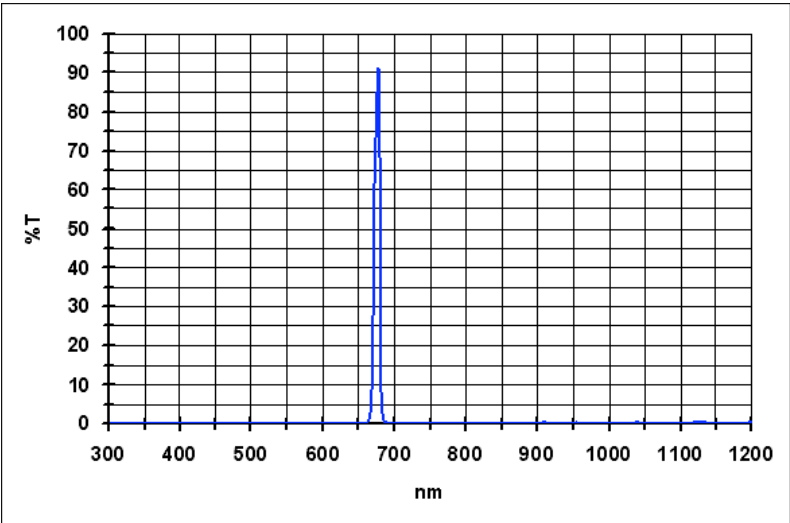
S-II
